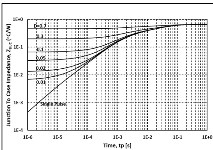
图. 23 热阻曲线
